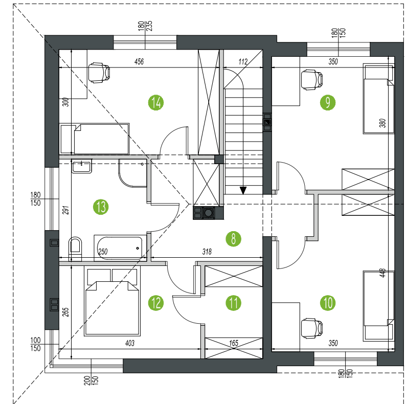
rzut piętra
